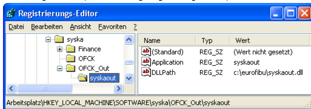
Abb. "Registrierungs-Editor"
